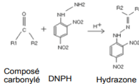
Figure 1 : Principe de chimisorption du formaldéhyde, réaction des composés carbonyles avec la DNP.
